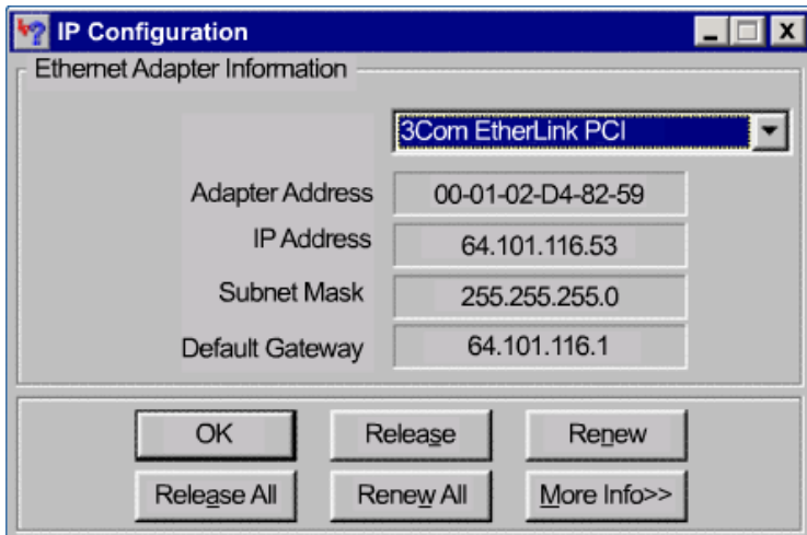
Fig. 5 – Comando winipcfg
