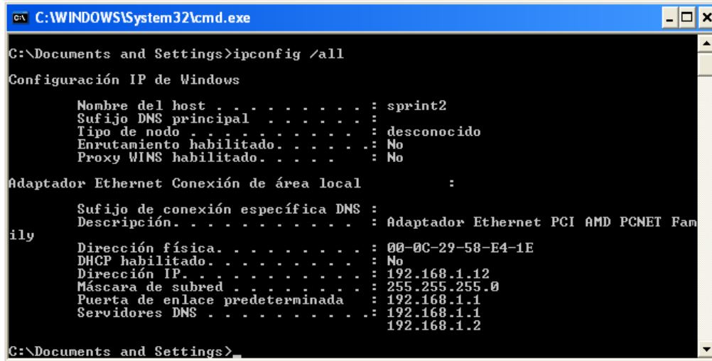
Fig. 4 – Comando ipconfig
